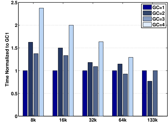
(a) D3Q19
